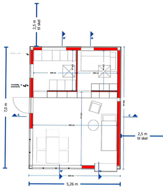
Grundplan 1:50
